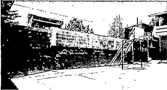
pintada de muro perimetral de 150 m2 e instacion de torta de piso de concreto de 7 cm de grosor de la cancha de basquetbol.
