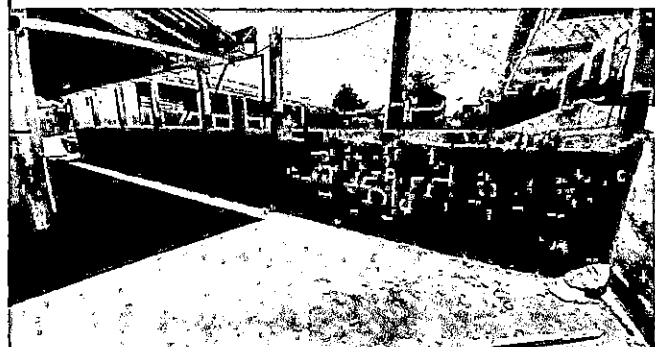
Instalacion de piso de concreto de 7 cm de grosor por 30 metros de longitud
